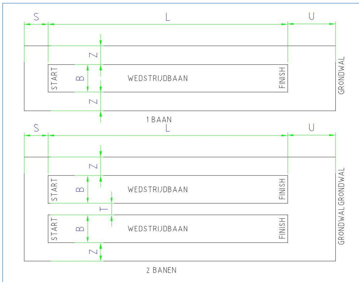
Figuur 1: Baanafmetingen
